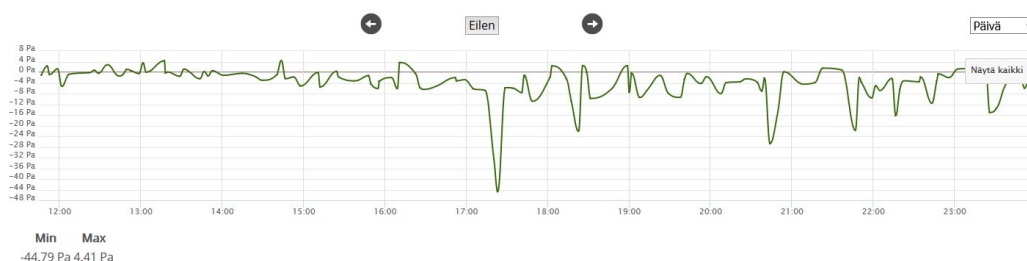
Kuva 6. Tuulen vaikutus mitattavaan paine- eroon
